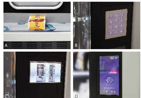
A - Tasca di prelievo maggiorata B - Tastiera illuminata C - Display grafico a colori, 480x272 pixel D - Interfaccia TABLET da 7"
